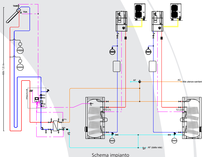
Schema impianto
